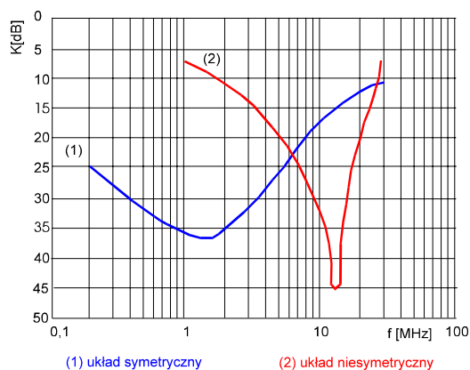
Charakterystyka tłumienności kondensatorów
