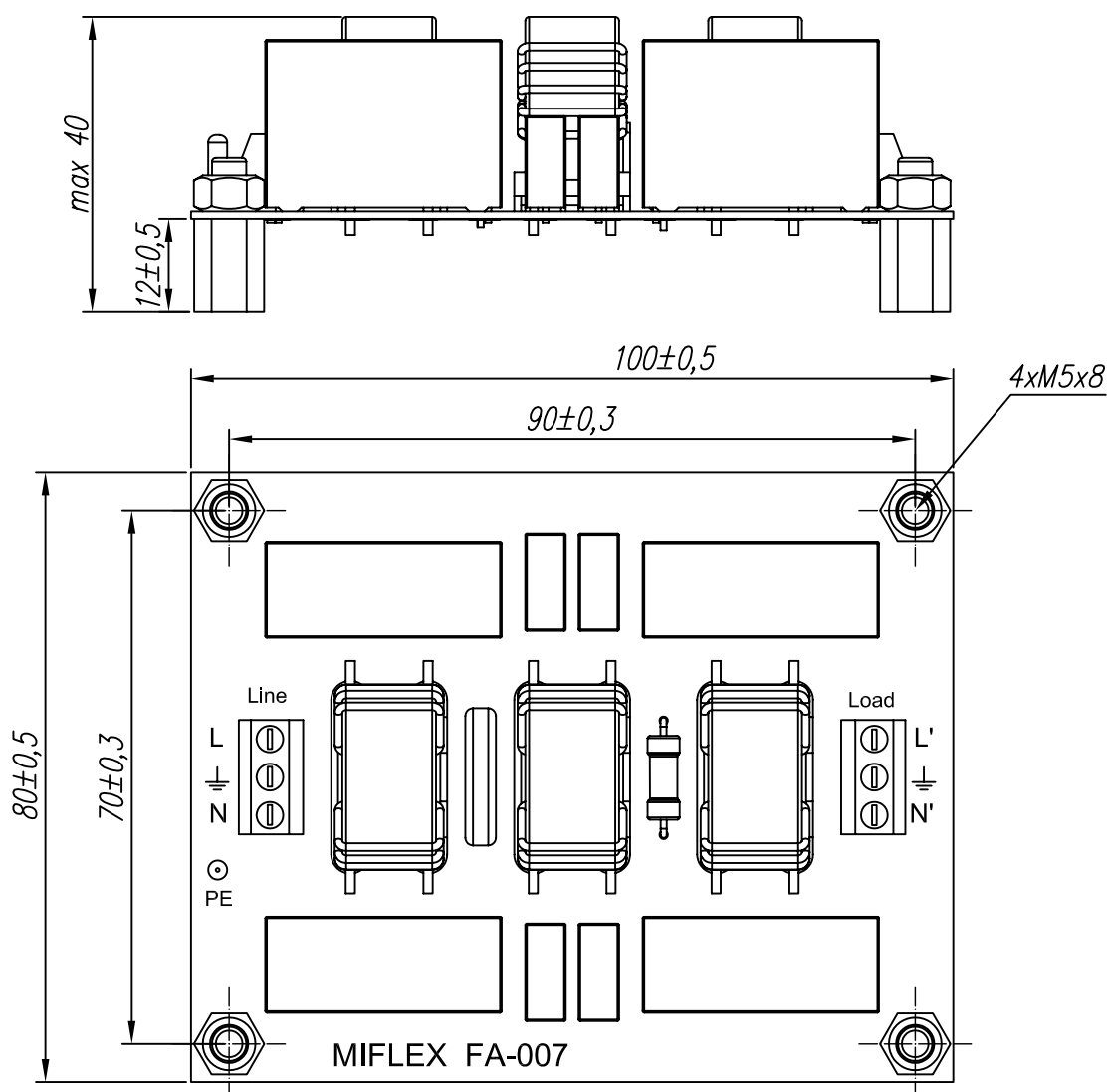
Podstawowe wymiary
